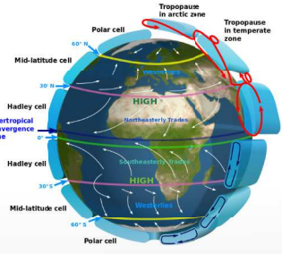
出典: http://commons.wikimedia.org/wiki/File:Earth_Globl_Circulation_-_en.svg
